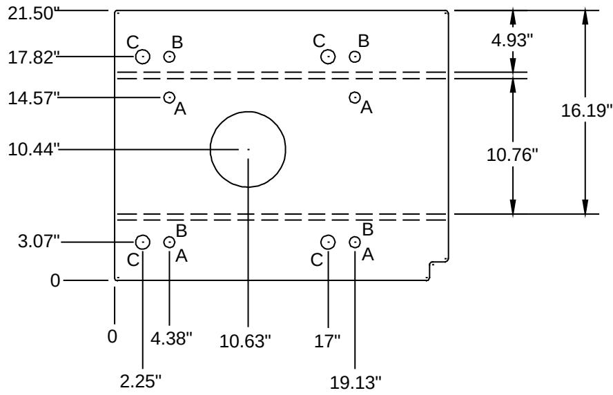
HOLE INDEX PER CRANE MODEL:
